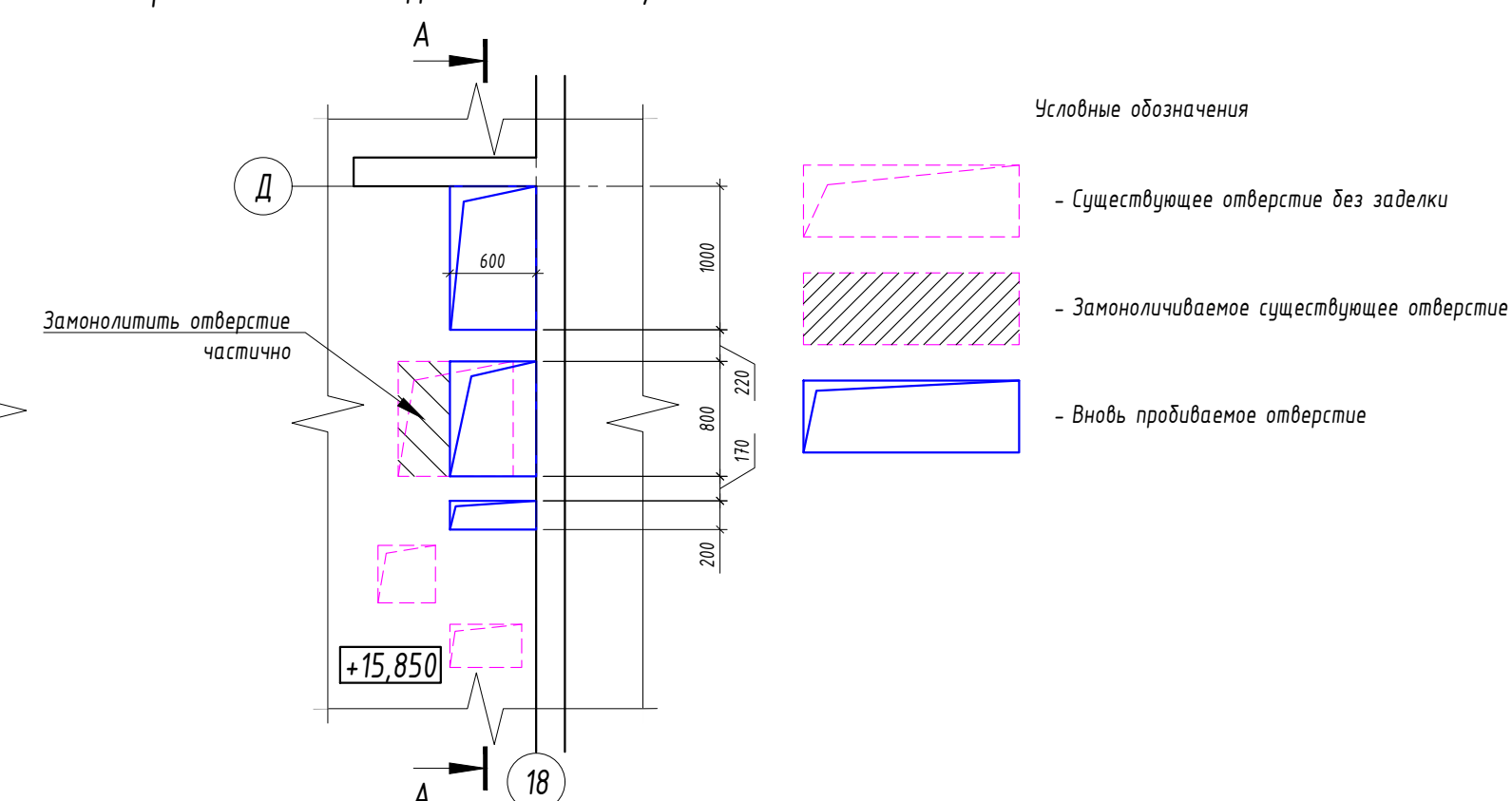
Фрагмент 1 в осях Д/18 на отм. +15,850
