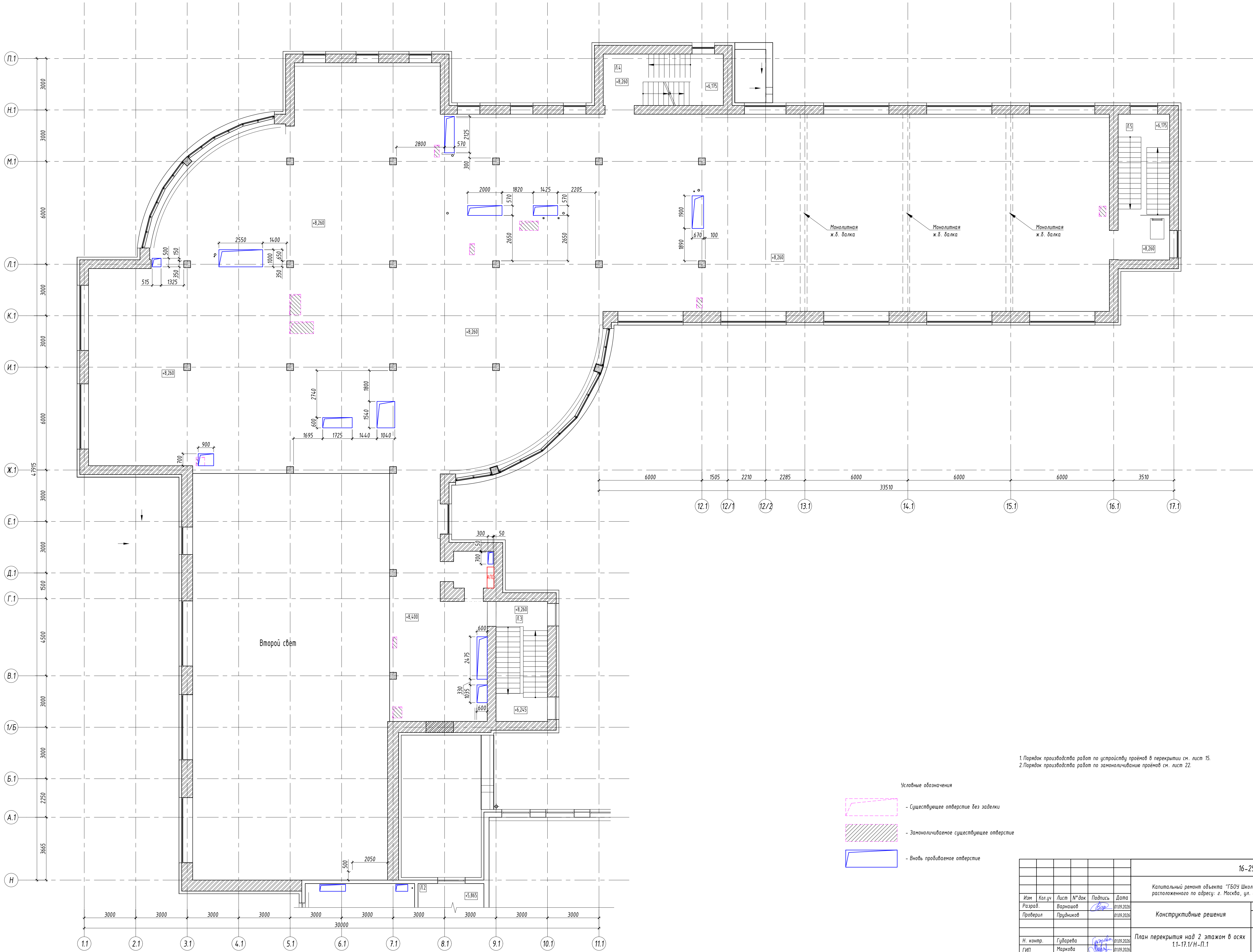
План перекрытия над 2 этажом в осях 1.1-17.1/Н-П.1
