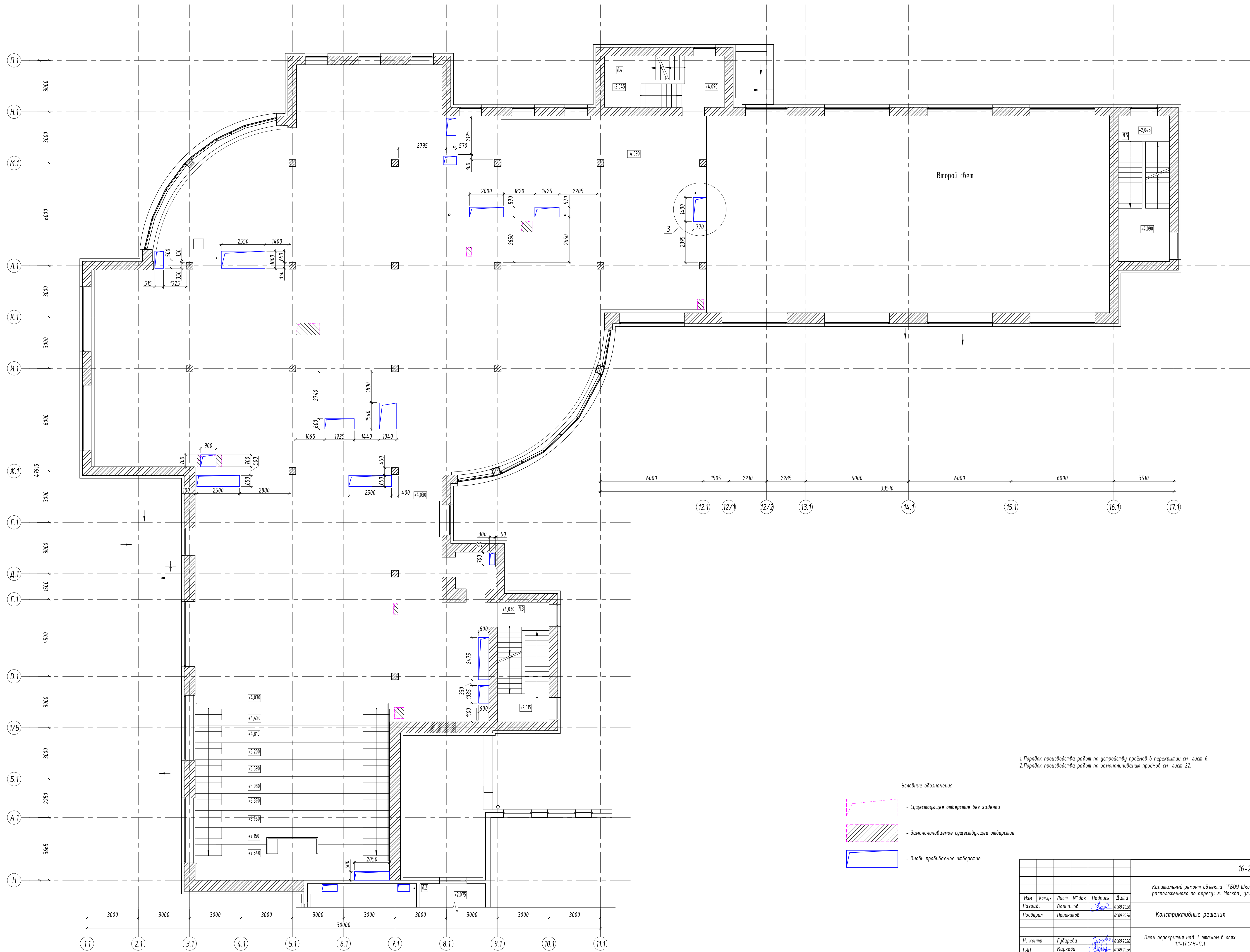
План перекрытия над 1 этажом в осях 1.1-17.1/Н-П.1
